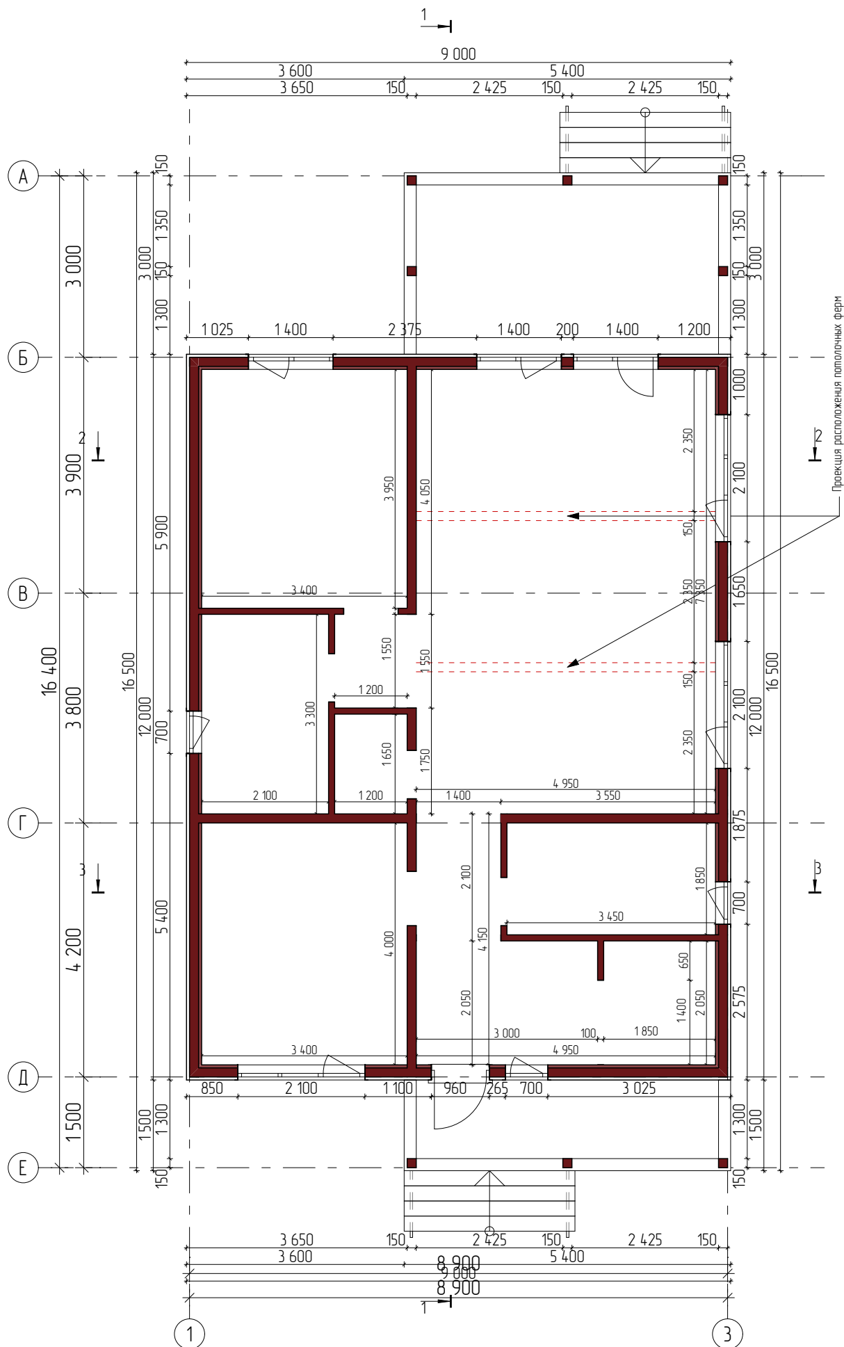
Детальный план 1-го этаж
